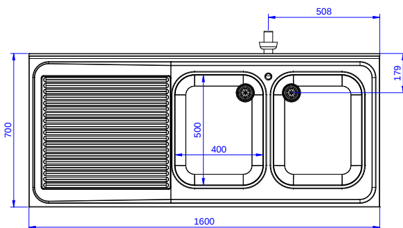
Boven aanzicht
